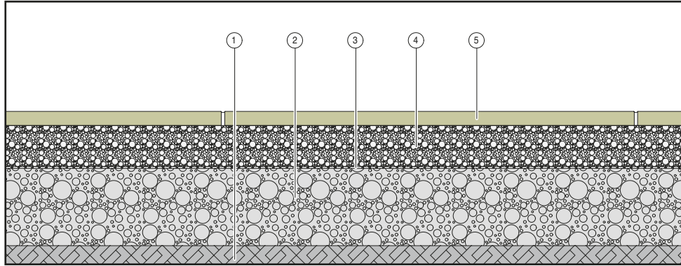
Gebundene Verlegung auf Drainagemörtel
